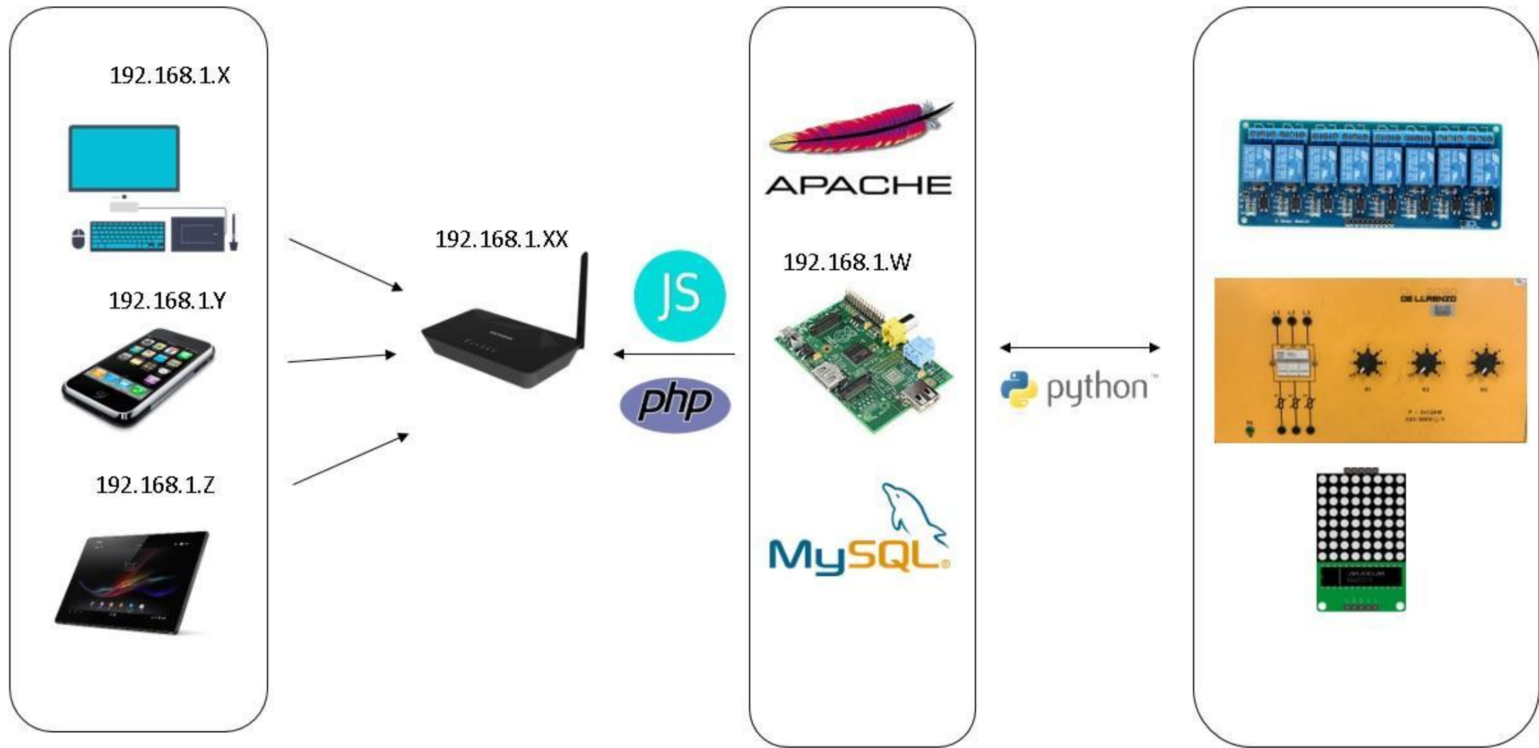
Diagrama de Bloques. Sistema de selección
