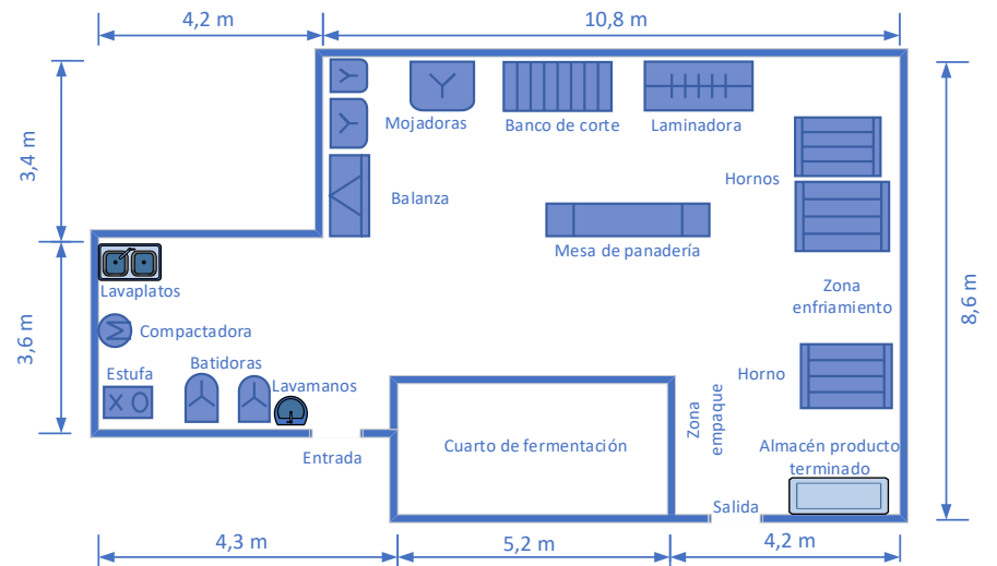
Distribución de planta propuesto
