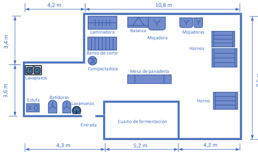
Distribución de planta actual
