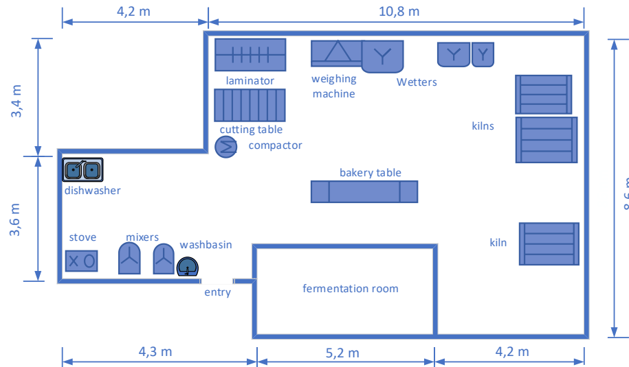
Actual Distribution Layout
