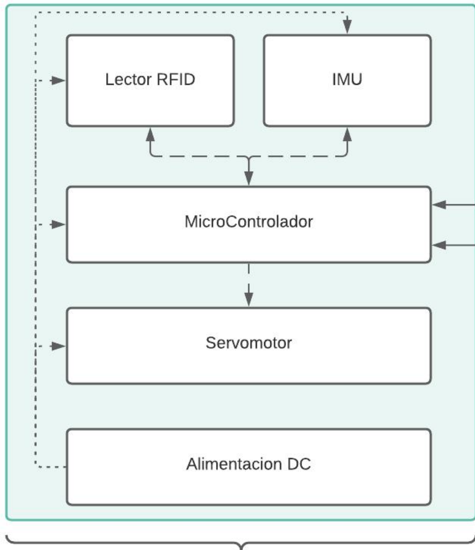
Sistema Radar
